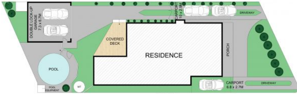
SITEPLAN
