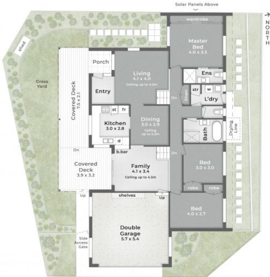
1:1 FLOOR PLAN & SITE PLAN
